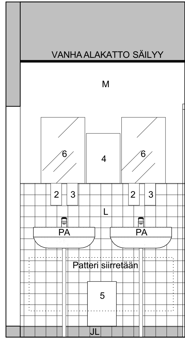
A-A Leikkaus 1:20
