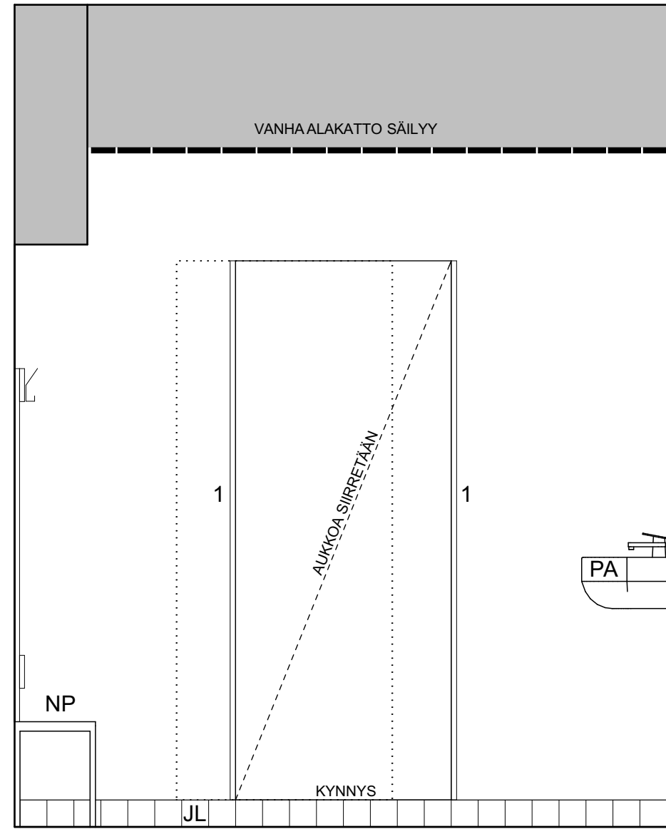
B-B Leikkaus 1:20
