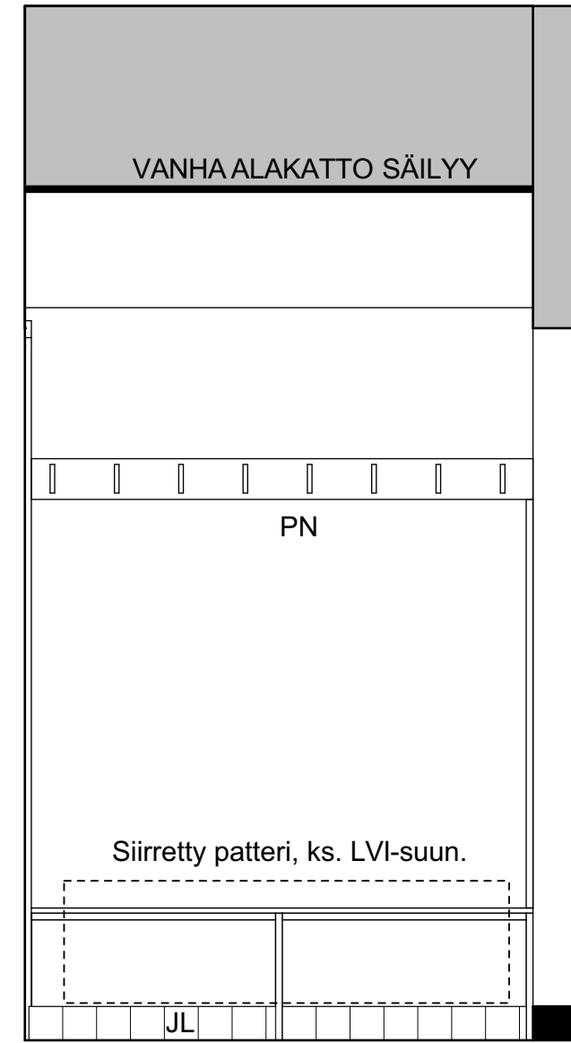
C-C Leikkaus (1) 1:20
