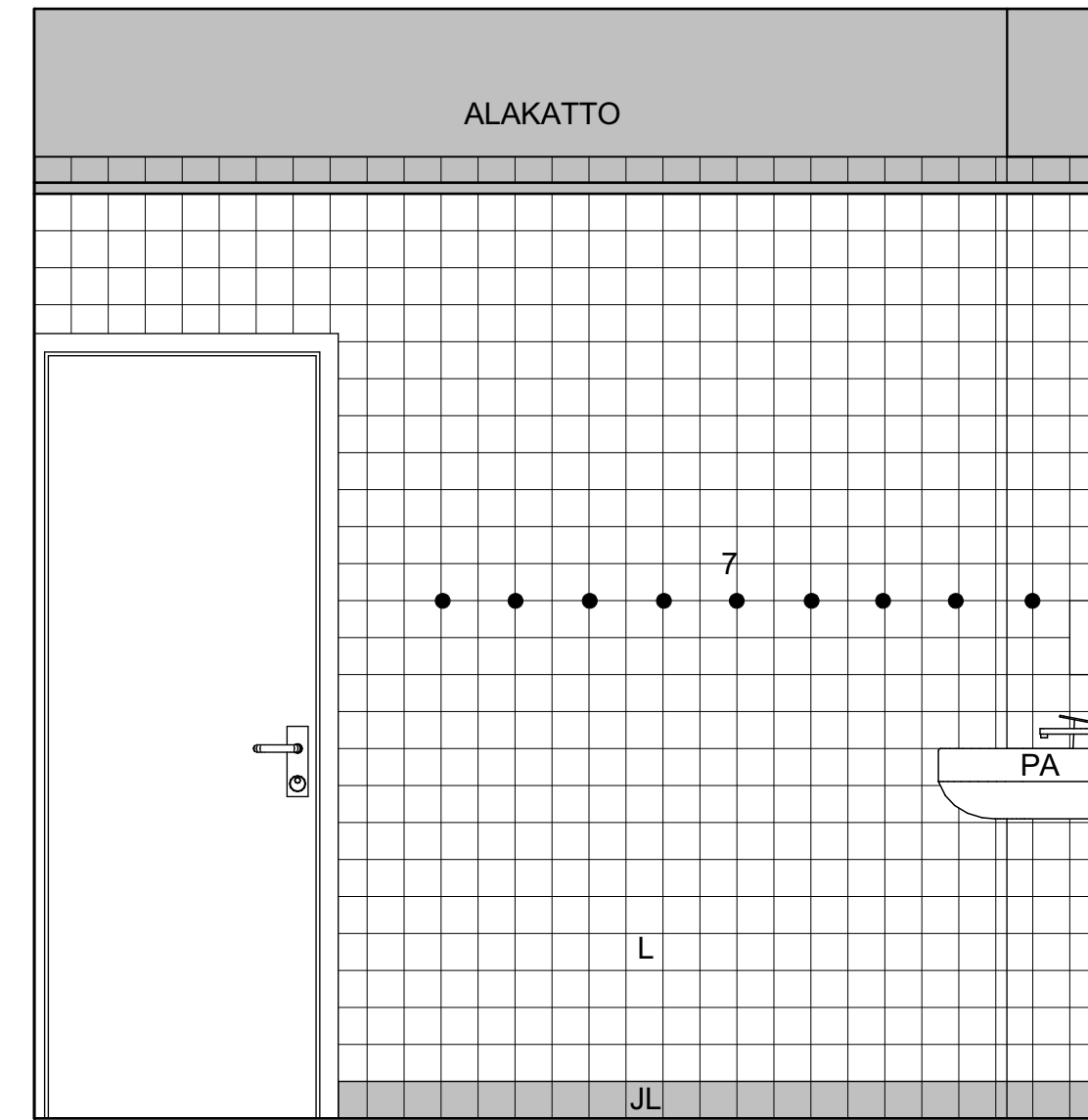
B-B Leikkaus 1:20
