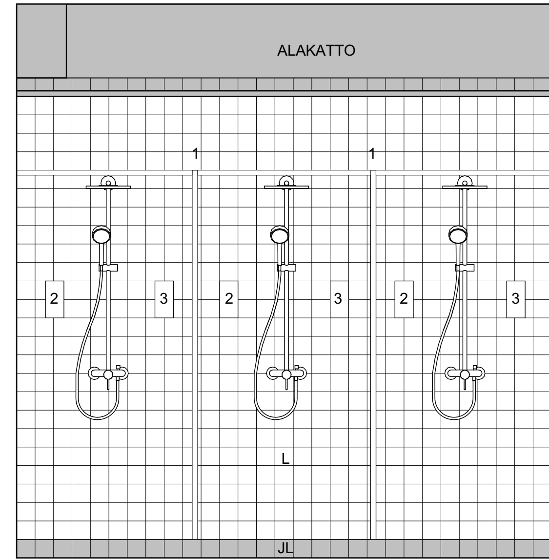
A-A Leikkaus 1:20
