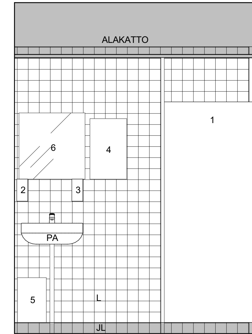
C-C Leikkaus (1) 1:20
