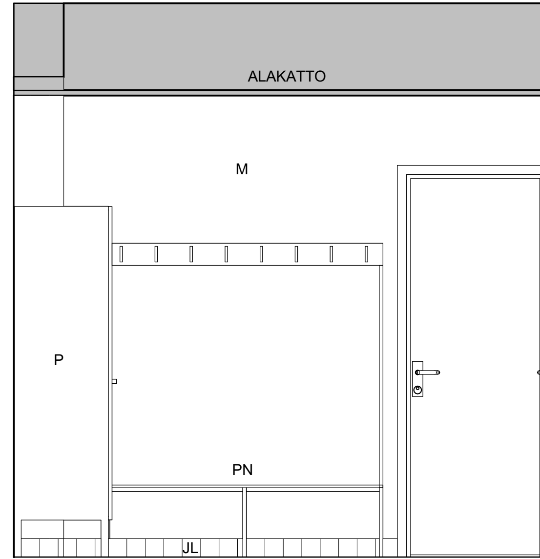
B-B Leikkaus 1:20
