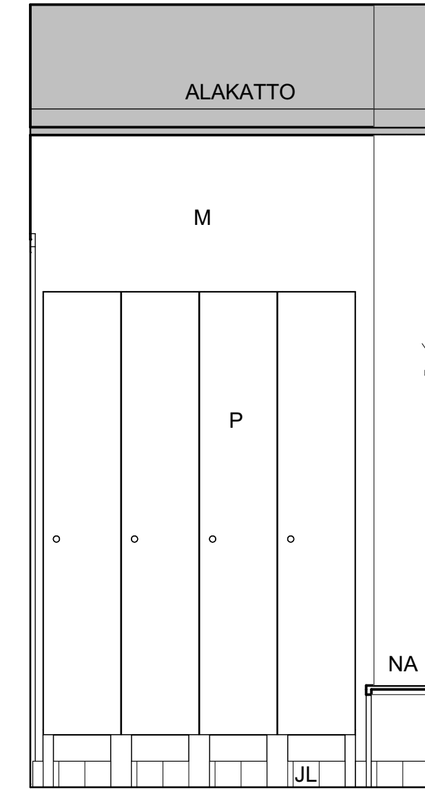
C-C Leikkaus 1:20
