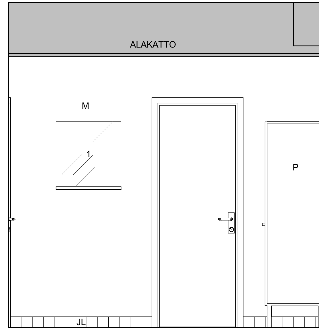
A-A Leikkaus 1:20
